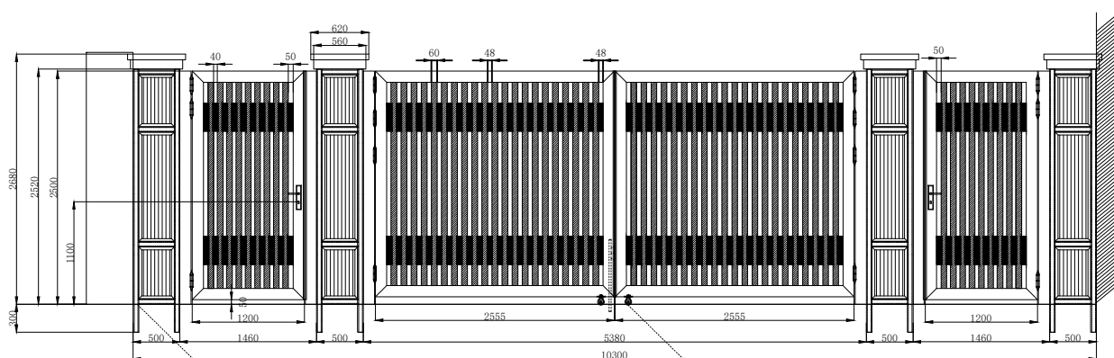
主视图
