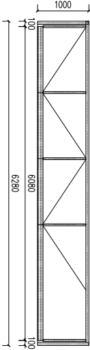
1D 框架顶面图
